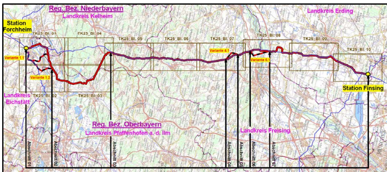
Abbildung 11: Übersichtsplan des Vorhabens mit Varianten (ohne Maßstab)
