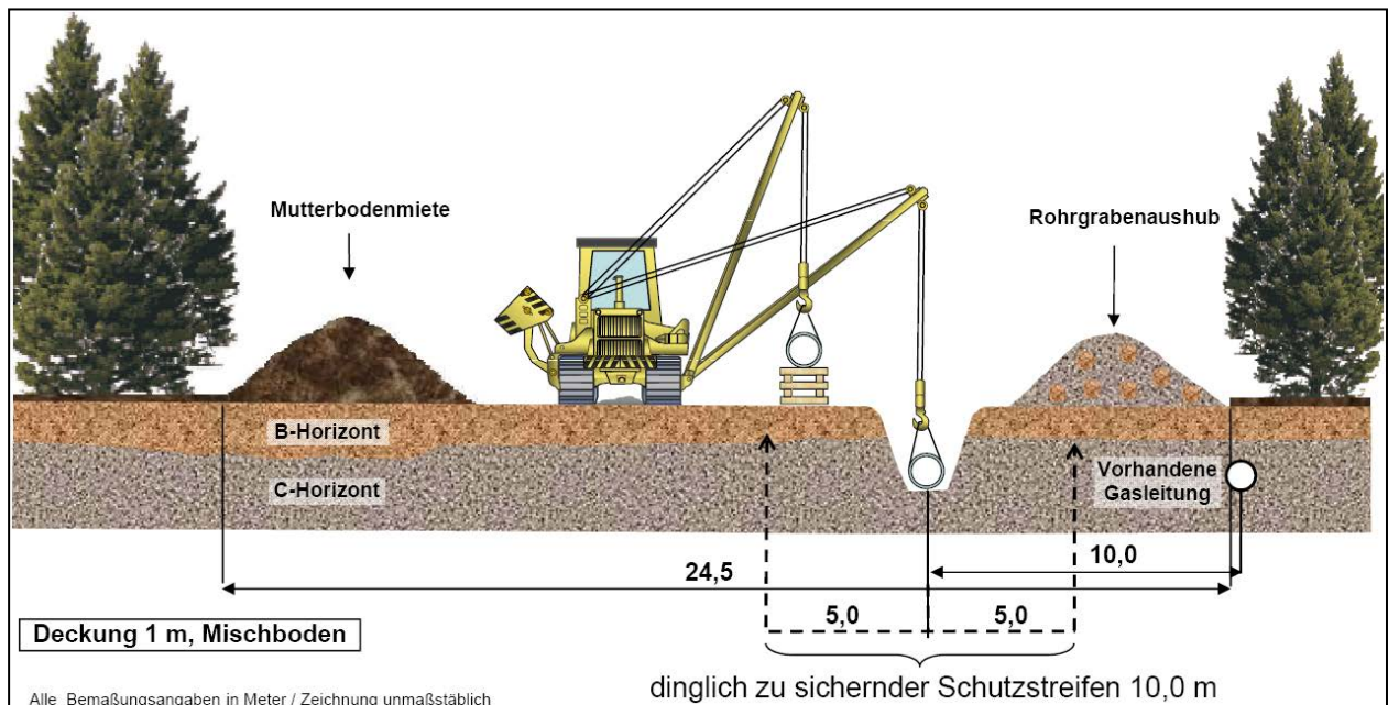
Abbildung 2: Regelarbeitsstreifen bei Leitungsverlegung mit Durchmesser DN 1000 in sensiblen Gebieten (Bsp. Wald) / Parallellage mit 10 m Achsabstand
