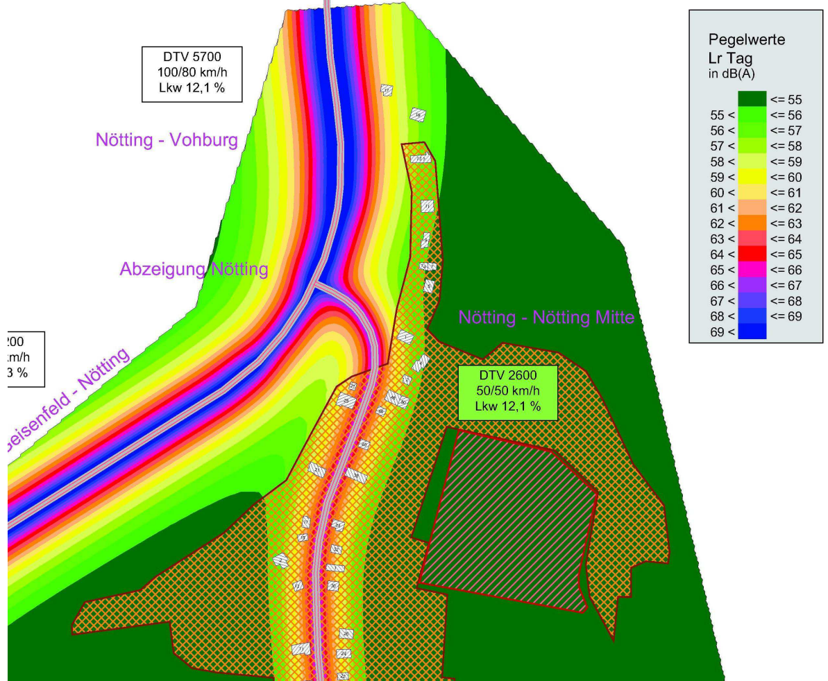
Abbildung 5-2: Rasterlärmkarte am Tag, Variante 2
